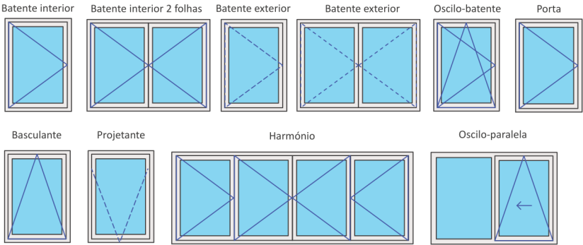
Sistema de câmara europeia com profundidade de aro de 67/73 mm
